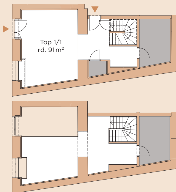
Grundriss des Geschäftslokals im Erdgeschoß und im Hochparterre, Top 1/1
